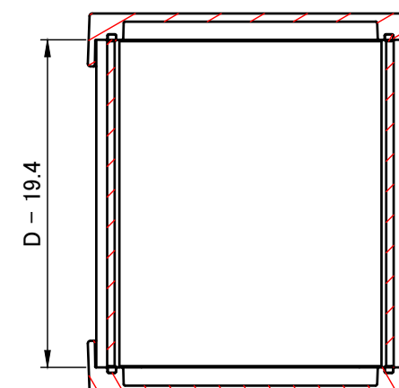
C-C ( 1 : 2.5 )
